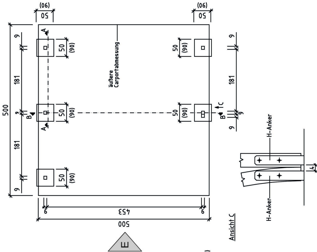
Grundriss
