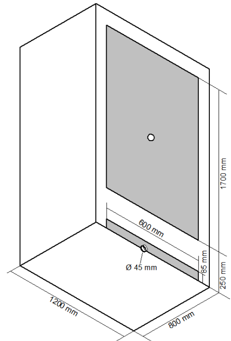
■ Anschlussmaße Korsika
