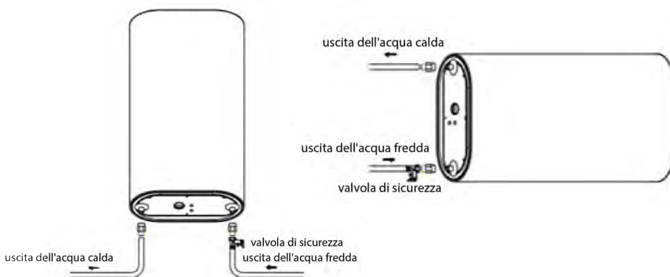
Figura 2: Installazione conforme
