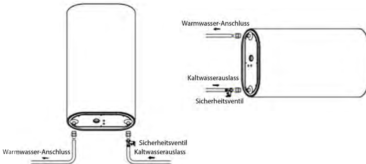
Abbildung 2: Konforme Installation
