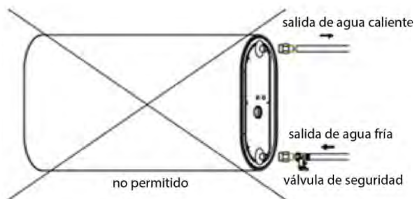
Figura 3: Instalación no conforme
