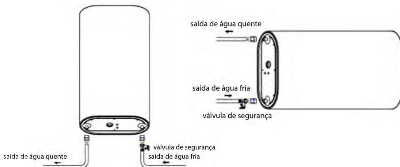
Figura 2: Instalação conforme
