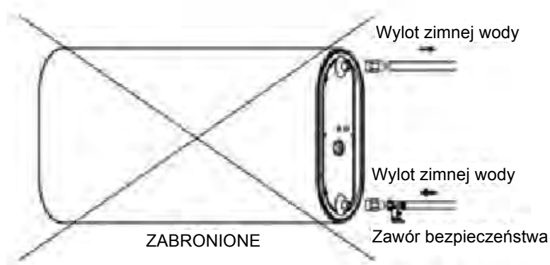
Rysunek 3: Instalacja niezgodna z przepisami
