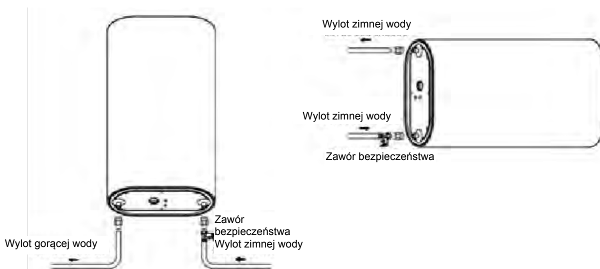
Rysunkiem 2: Instalacja zgodna z przepisami
