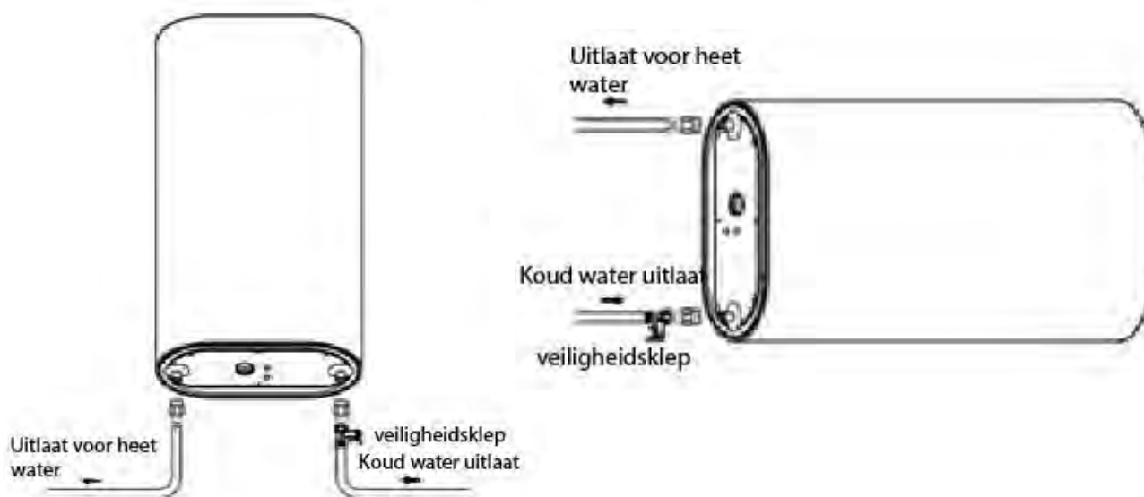
Figuur 2: Conforme installatie
