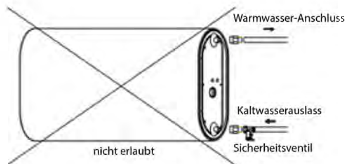
Abbildung 3: Nicht-konforme Installation
