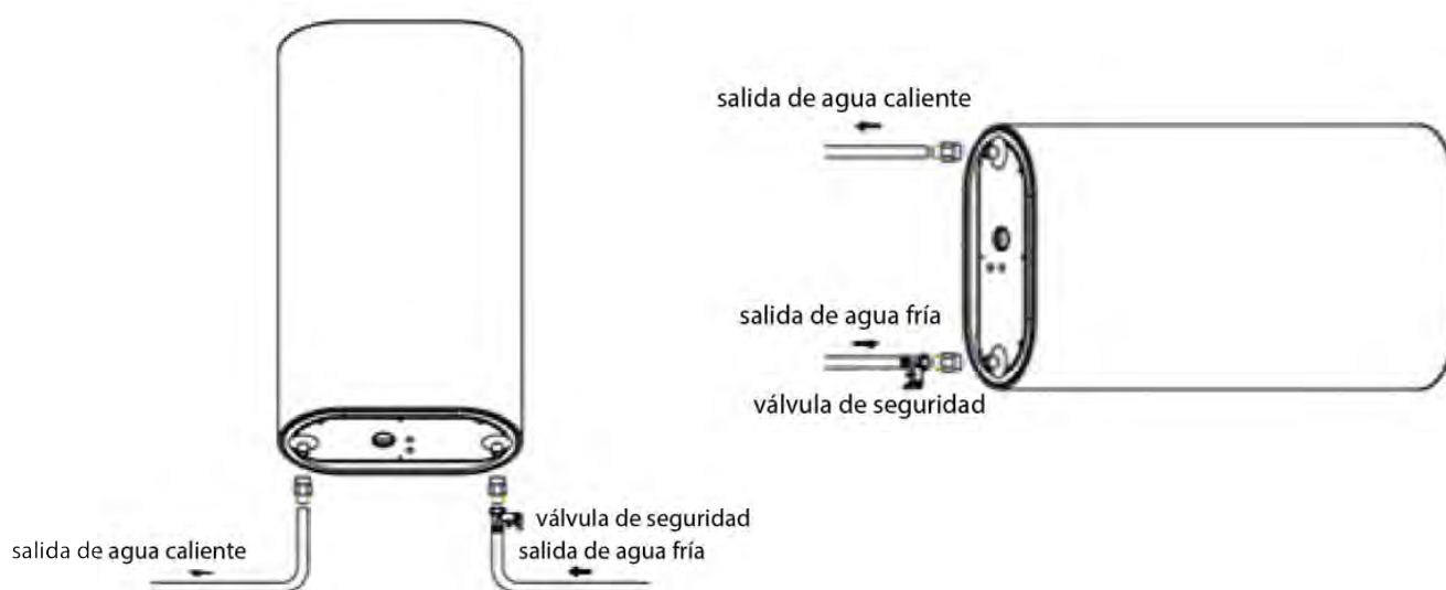
Figura 2: Instalación conforme
