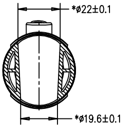
截面 A-A
