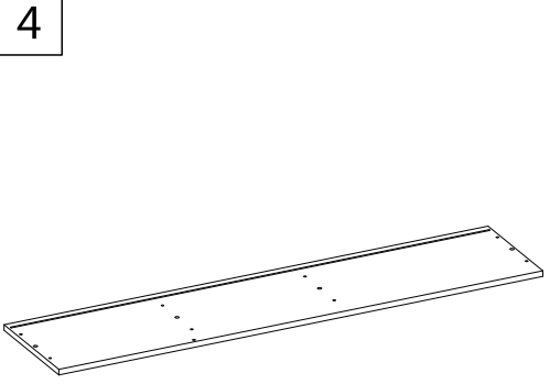
1034*239*12mm 1PC
