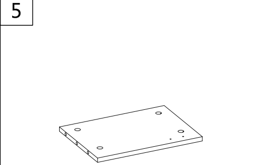
1034*239*12mm 1PC
